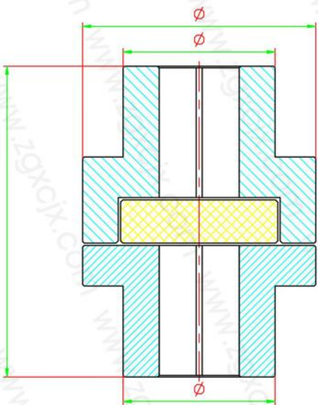
外形尺寸
